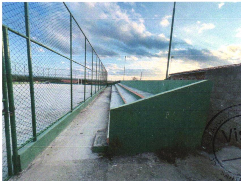
Foto 02 – PISO EM CONCRETO 20 MPA PREPARO MECÂNICO, ESPESSURA 7CM. AF_09/2020
